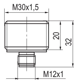
Габаритный чертеж
